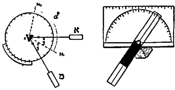
ציור 1. גוניומטר-הסנסע ציור 2. גוניומטר-ההחזרה
